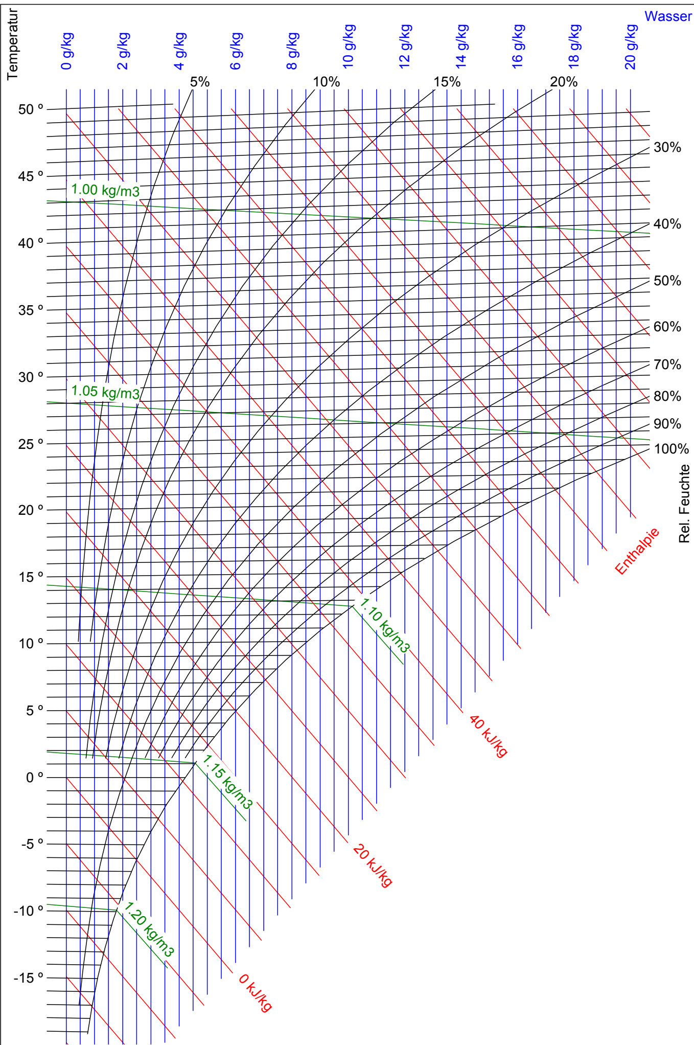
Mollier-h-x-Diagramm für feuchte Luft - Druck 0.908 bar (900.000 m / 6.000 °C / 80.000 % rF)
