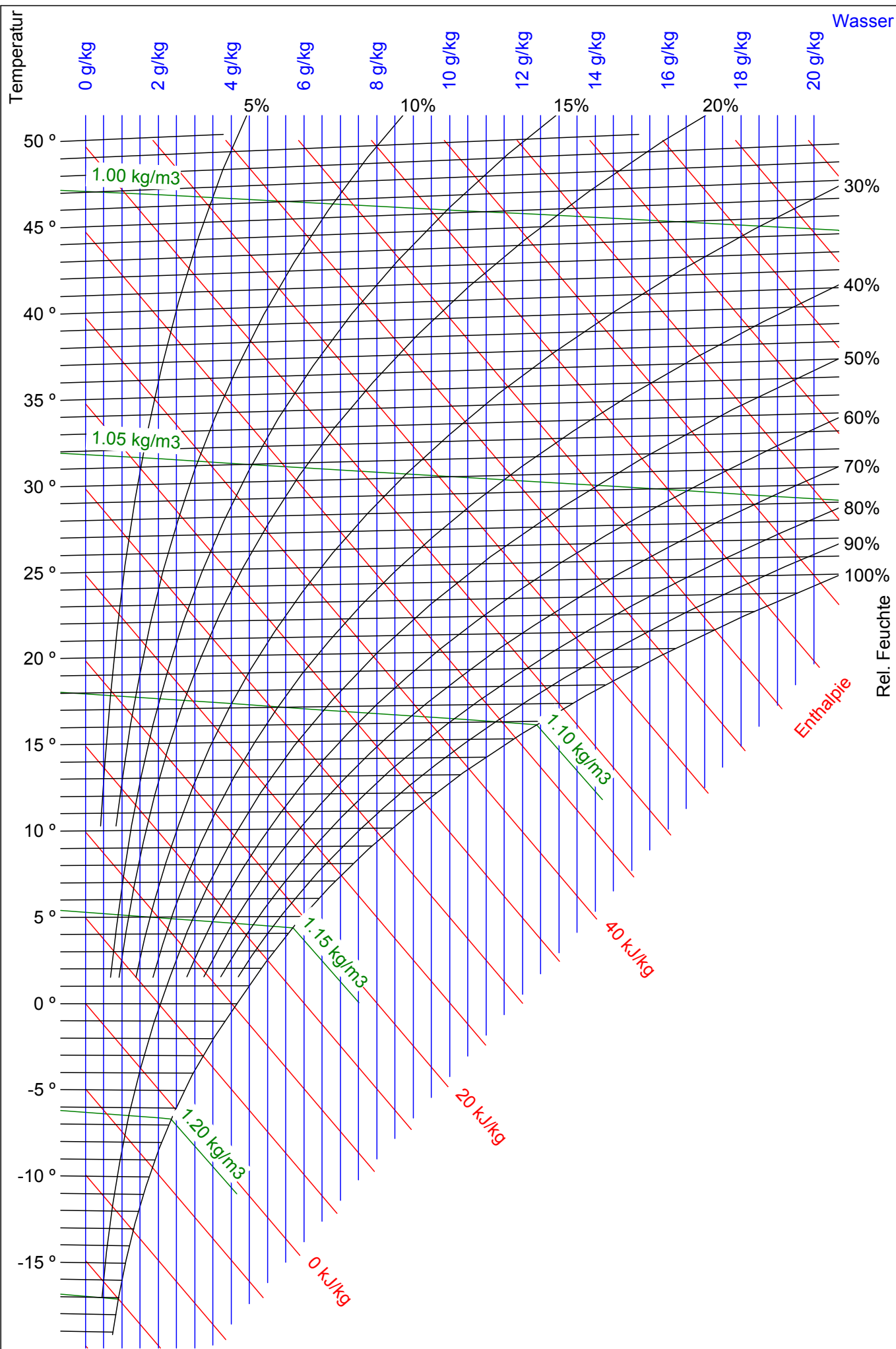
Mollier-h-x-Diagramm für feuchte Luft - Druck 0.919 bar (800.000 m / 7.000 °C / 80.000 % rF)
