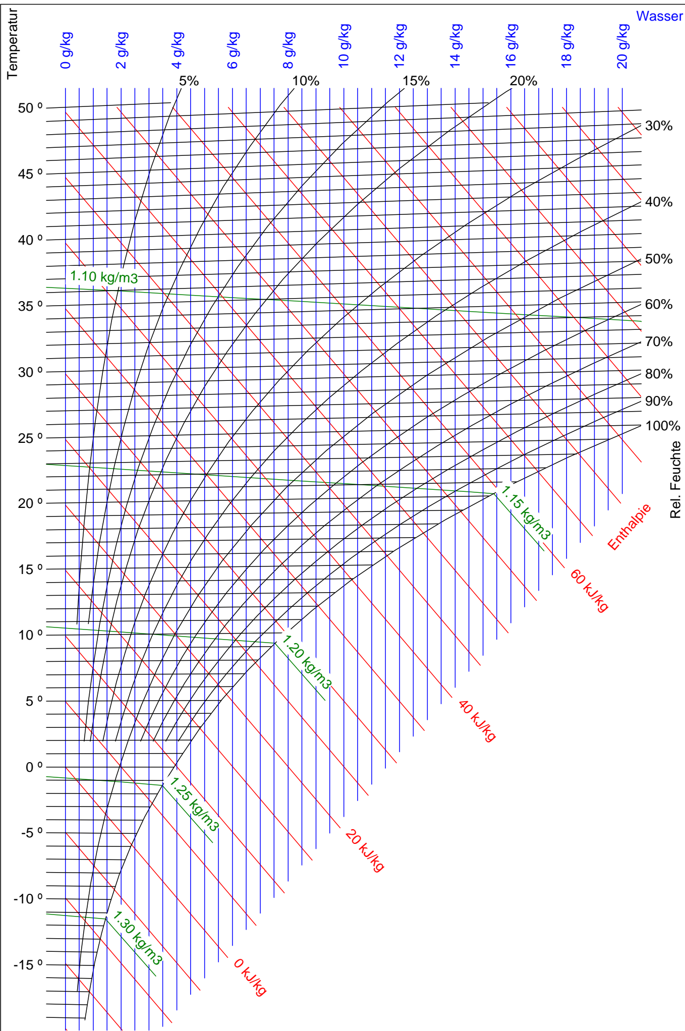
Mollier-h-x-Diagramm für feuchte Luft - Druck 0.977 bar (300.000 m / 10.000 °C / 80.000 % rF)
